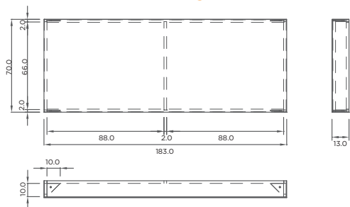
Letreiro Premium P vistas ortográficas do módulo convexo
