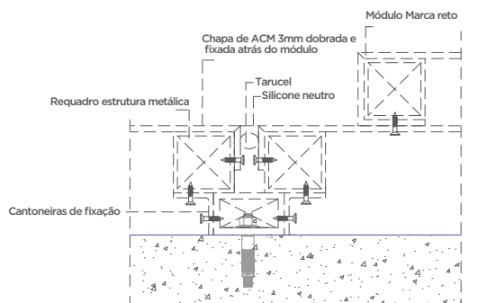
Detalhamento fixação entre os módulos
