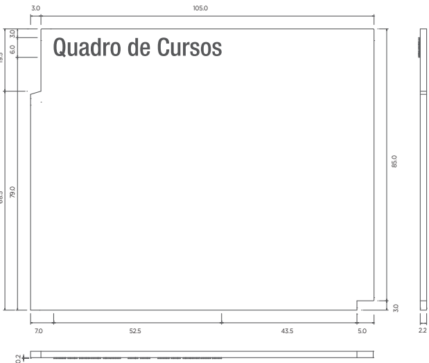
Chapa Acrílica vistas ortográficas
