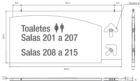
Peças Montadas vistas ortográficas
