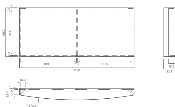
Letreiro Premium G vistas ortográficas do módulo convexo
