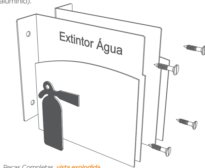
Peças Completas vista explodida
