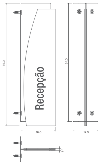
Peças Montadas vistas ortográficas
