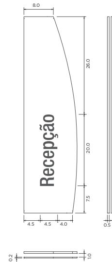
Chapa Metálica vistas ortográficas do verso
