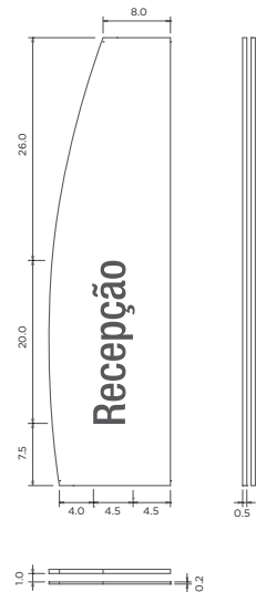
Chapa Metálica vistas ortográficas da frente
