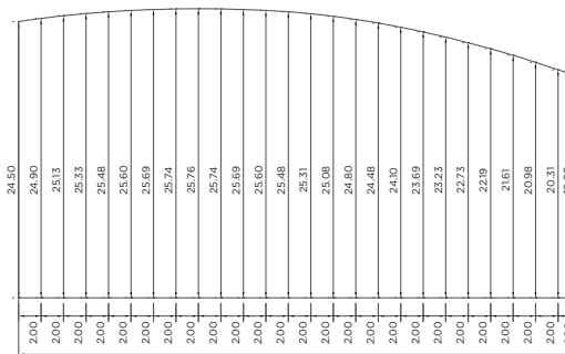
Chapa Metálica flecha
