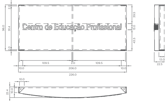
Letreiro Premium G vistas ortográficas do módulo info. adicional
